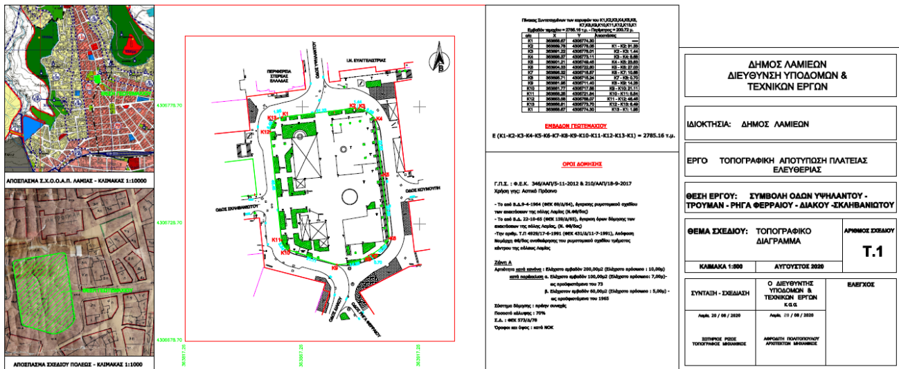
Εικόνα 1: Τοπογραφικό Διάγραμμα πλατείας Ελευθερίας (επισυνάπτεται στο Παράρτημα)
